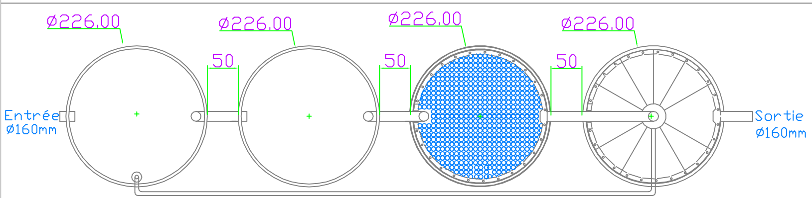
Vue de dessus
